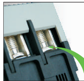
клеммы подключения с напайкой контактов
